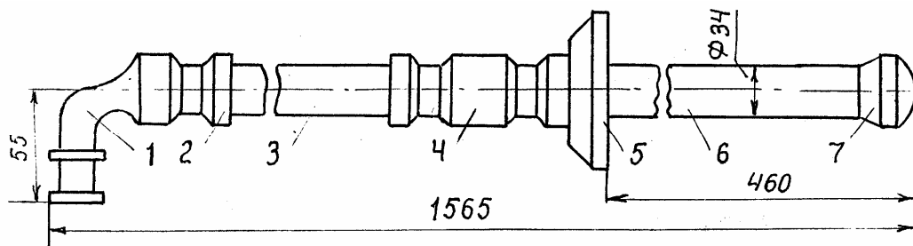
Рис.4. Оперативная штанга типа ШР-10 на 10 кВ
