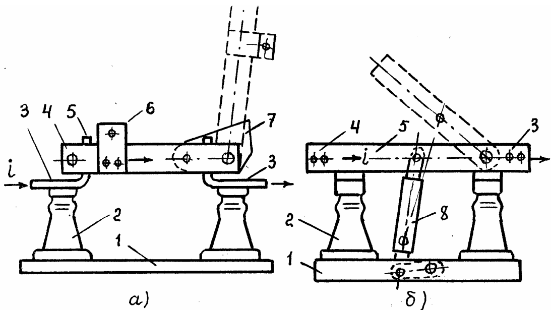
Рис.1. Конструктивные схемы разъединителей вертикально-поворотного типа: 1 – рама; 2 – опорный изолятор; 3 – вывод для присоединения подводящих проводов (шин); 4 – нож (подвижный контакт); 5 – неподвижный контакт; 6 – ушко для оперативной штанги; 7 – упор, ограничивающий поворот ножа; 8 – изоляционная тяга
